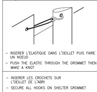
FIG. I BANDE ANTI-VENT / WINDSECURE KIT OPTIONNEL / OPTIONAL
